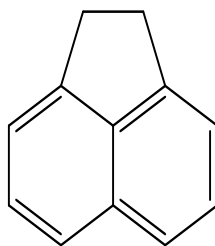
Acenaphthene
